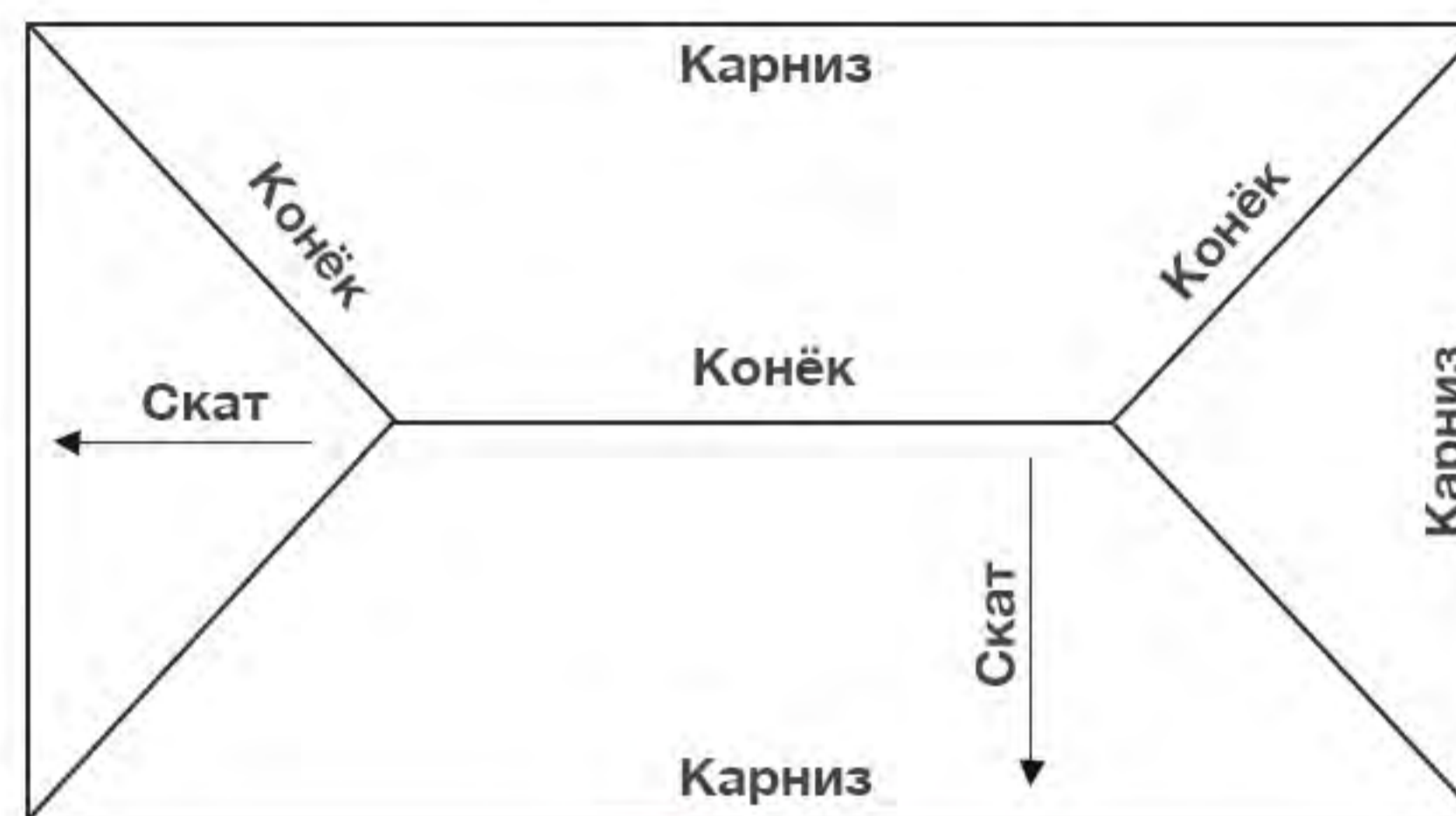
2. Четырёхскатная крыша
